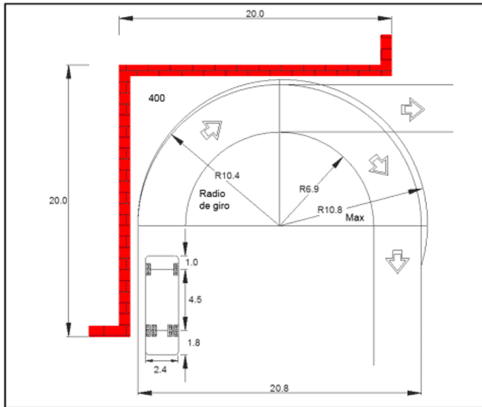
Figura 2. Radio de giro 12.20 -12.56 m para una superficie de 400 m 2 , en esquina.
