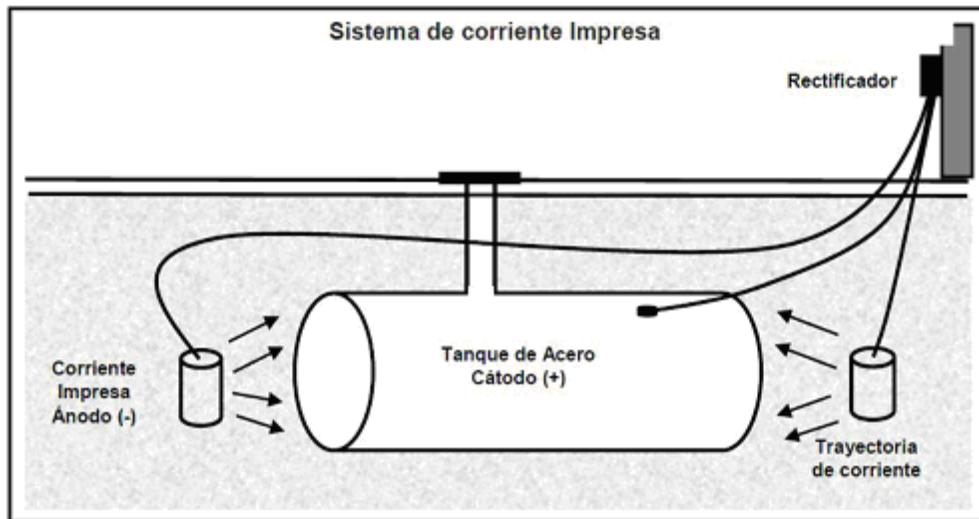
Figura 2. Sistema de protección catódica por corriente impresa
