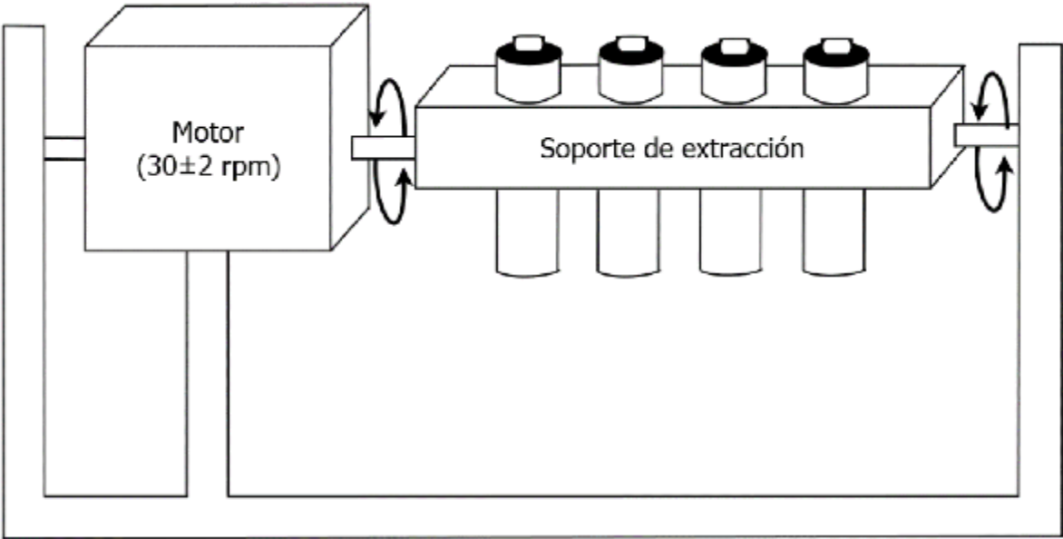
Figura C.1 Aparato rotatorio de agitación MÉTODO 1312
